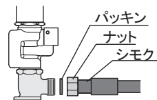
❗ 配管接続部を清掃する
